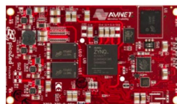
Avnet PicoZed™
